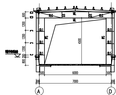
D~A轴墙面线条立面图
