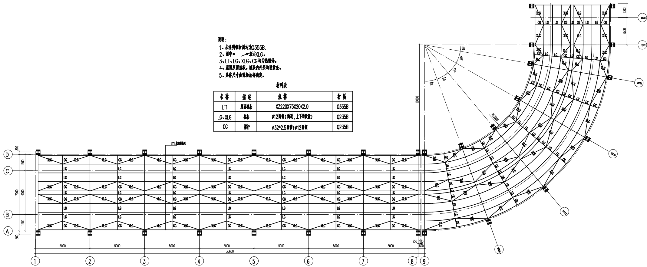
屋面拉条平面布置图 1:150
