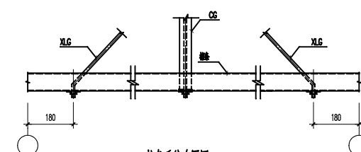
拉条系统布置图
